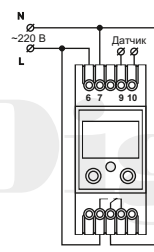
Схема подключения
