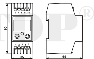
Габаритные размеры
